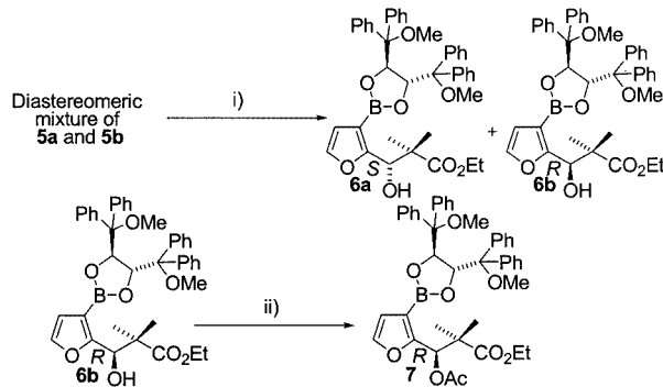
Scheme 1. i) 1 M HCl, THF, room temp., 15 min, 98%; ii) Ac 2 O, pyridine, reflux, 2 h, 82%
